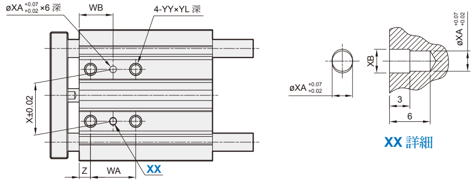
背面圖
