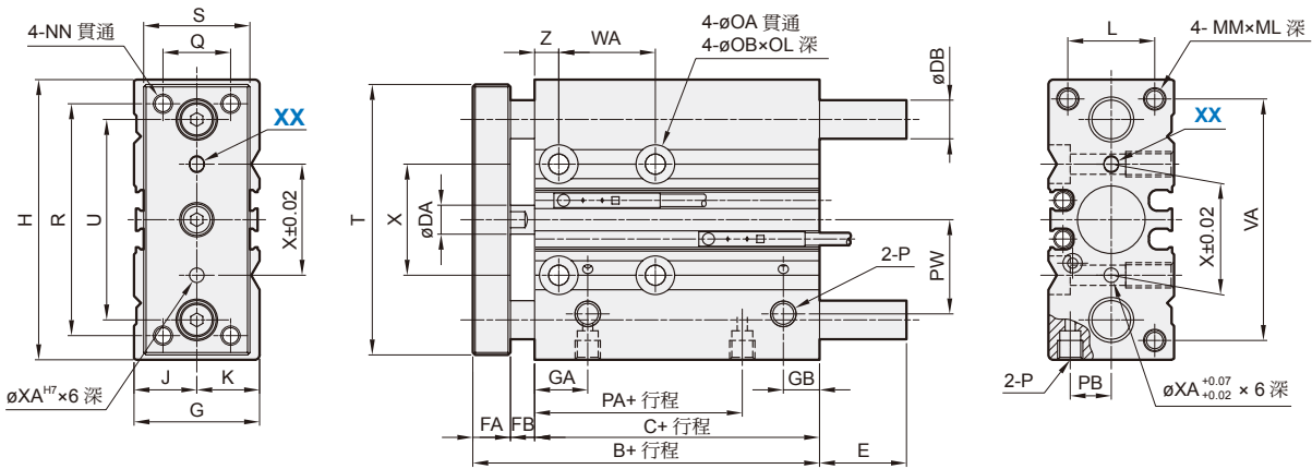
背面圖
