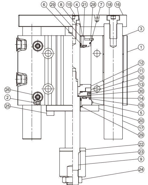
ø40~ø63
