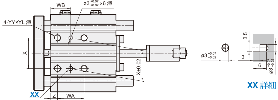
背面圖
